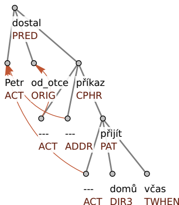
Fig. 2. The (simplified) dependency tree for the sentence Petr dostal od otce příkaz přijít domů včas ‘Peter was given the order from his father to come home on time’.
